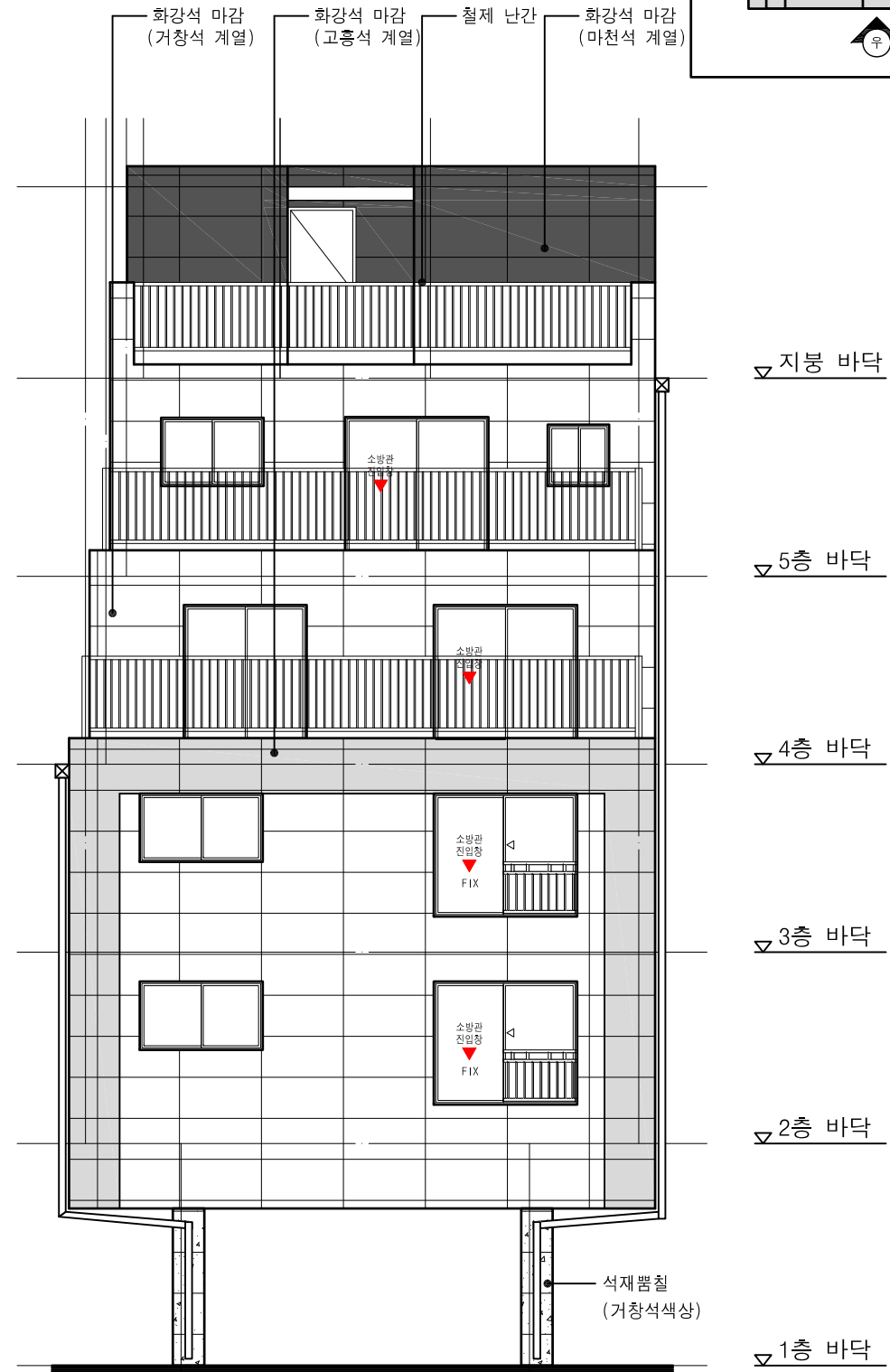
정 면 도 SCALE : A3 : 1/100
