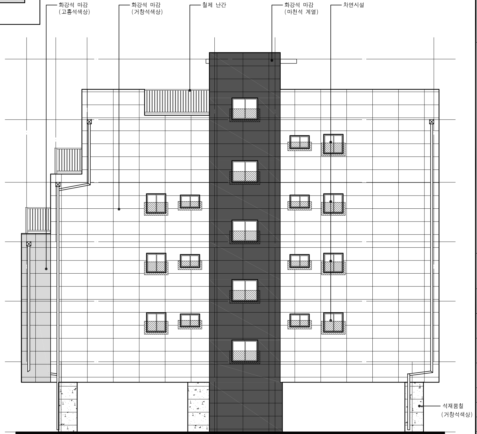
우 측 면 도 SCALE : A3 : 1/100
